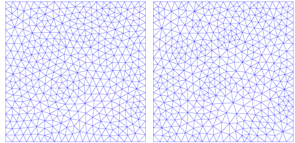
(c) ODT smoother I (d) CVT smoother I
